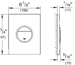
Nova Cosmopolitan 38 765 000 / 38 765 SH0
